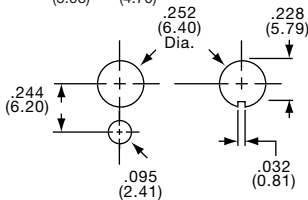
Horizontal Actuation
